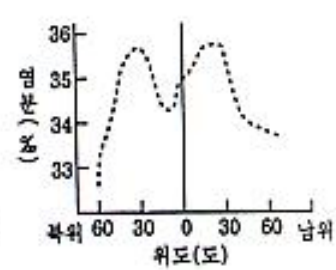
(다) 해수 표면의 염분 분포
